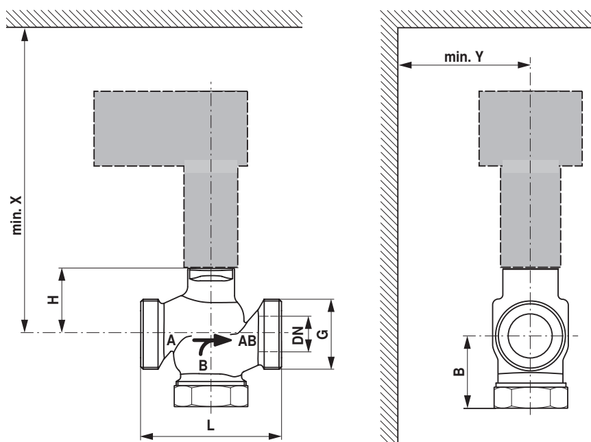
Rysunki wymiarowe
