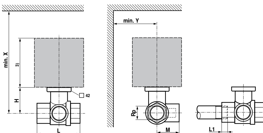
Rysunki wymiarowe
