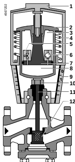
Zawór otwarty
