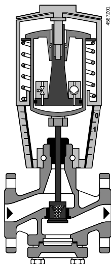
Zawór zamknięty
