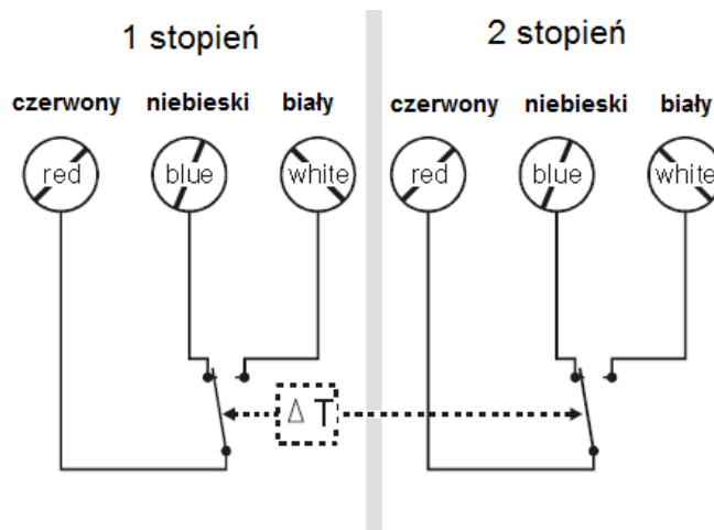
Rys. 4. Okablowanie T6120B1003
