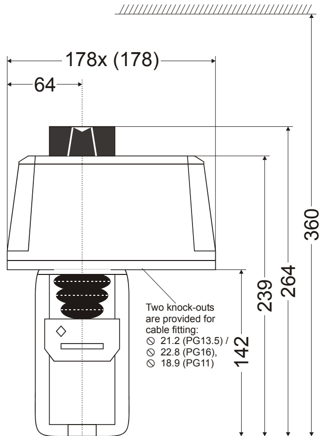
Rys. 4. ML6421A, ML7421A (w mm)
